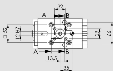
SEZIONE A-A SECTION A-A
